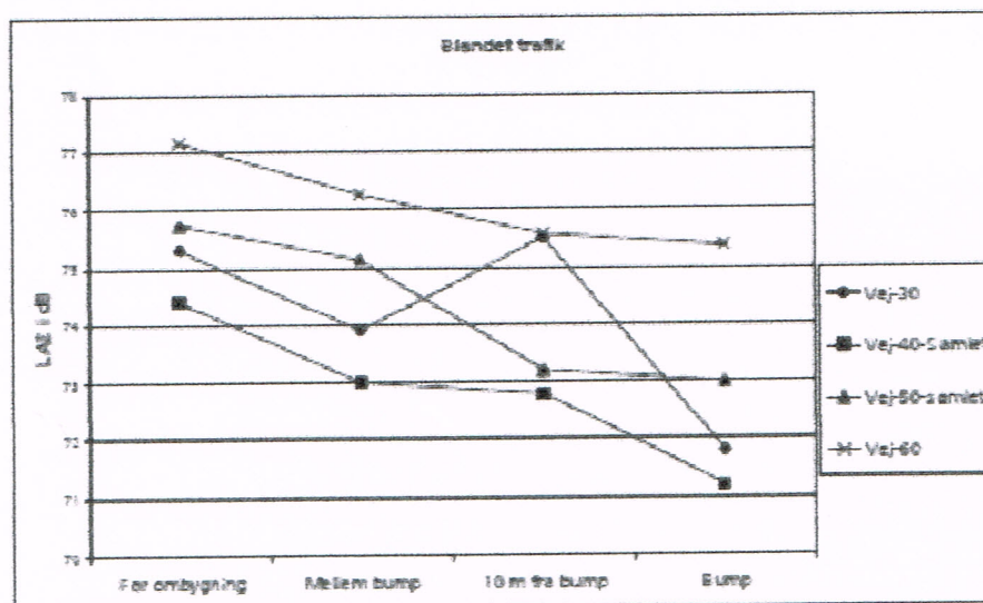
Figur 6.1: Støj ved bump på veje med skiltet hastighed 30km/t, 40 km/t, 50km/t og 60 km/t
