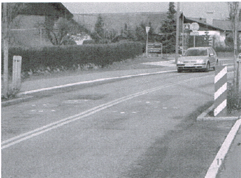
Figur 5.2: Pukkelbump på Gavnøvej i Næstved
