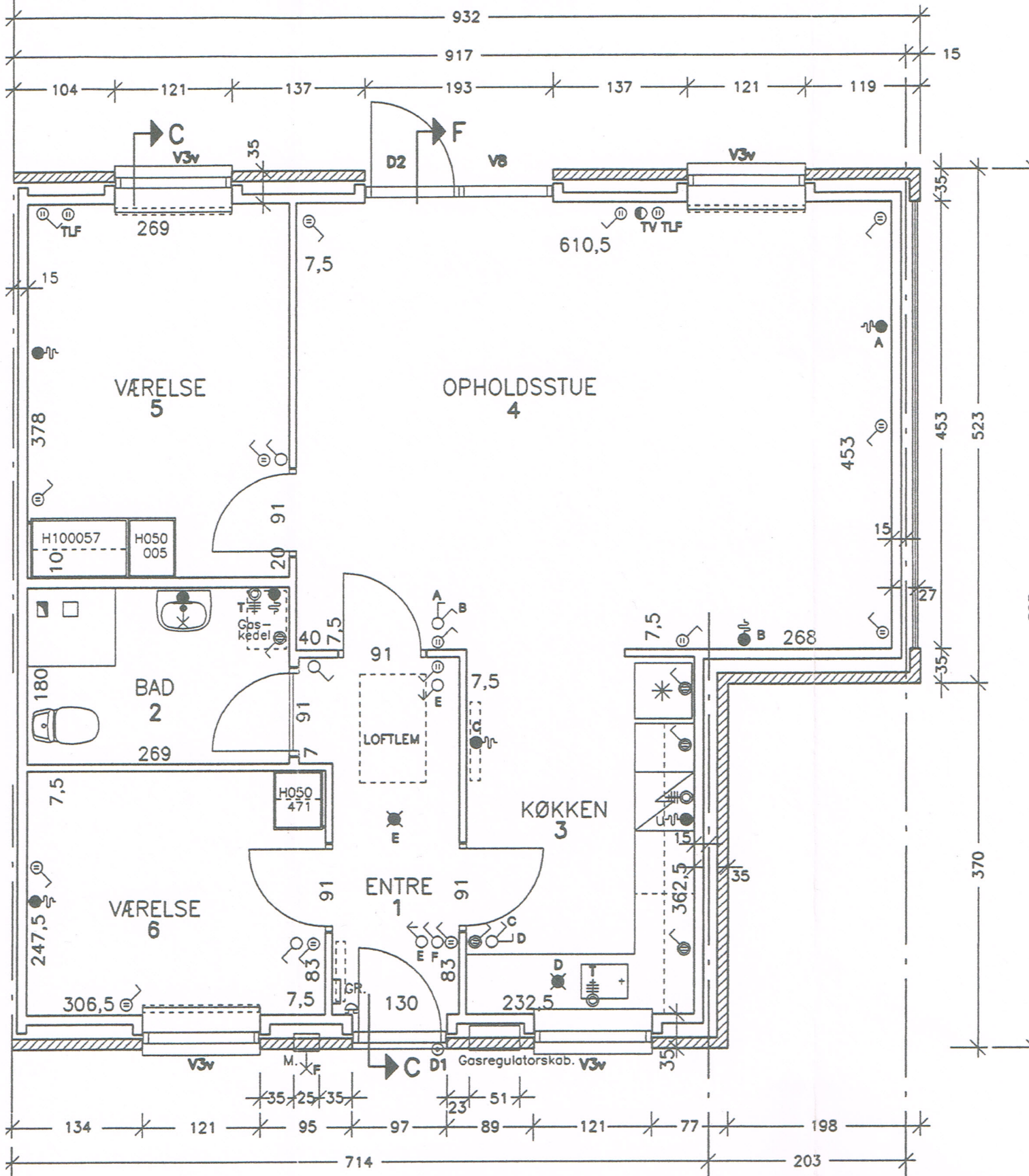
PLAN TYPE D - MÅL 1:50
